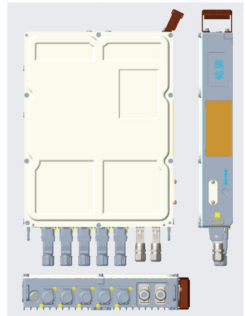
3kW Power module
